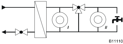
MOD 2: Погодозависимое управление температурой подающей (вторичной) с управлением питьевой водой с помощью управляющего клапана во вторичном контуре
