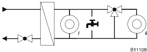
MOD 1: Погодозависимое управление температурой подающей (вторичной) с дополнительным управляющим клапаном во вторичном контуре для повторного нагрева
