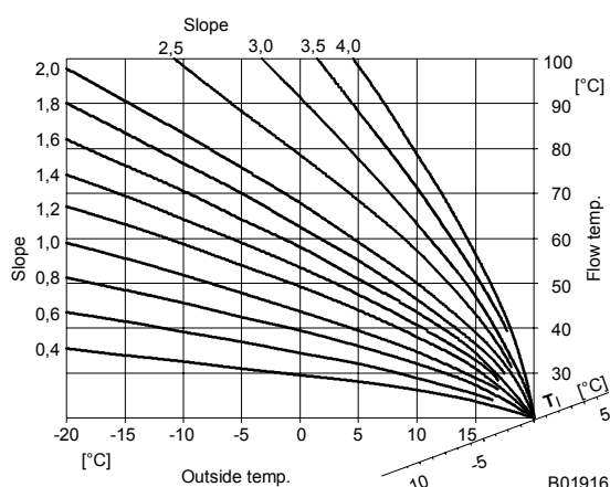
Характеристика отопления для базовой точки T_1 = 20\text{ °C}
