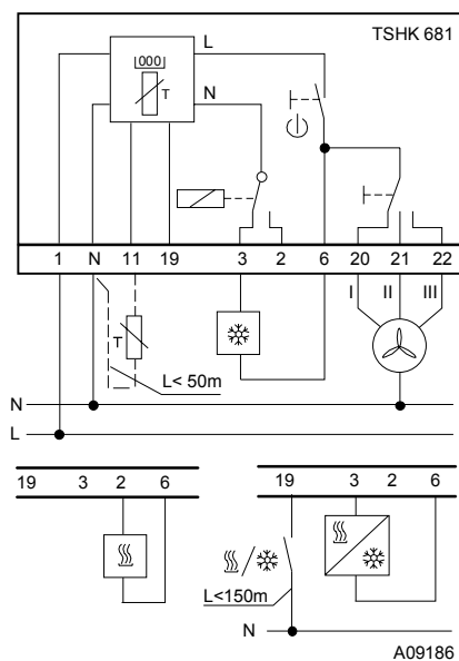
Схема подключения
