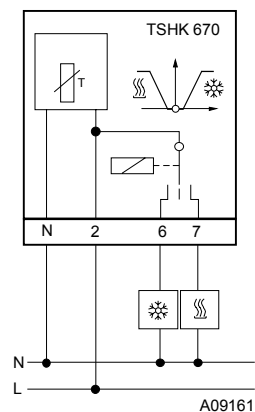
Схема подключения
