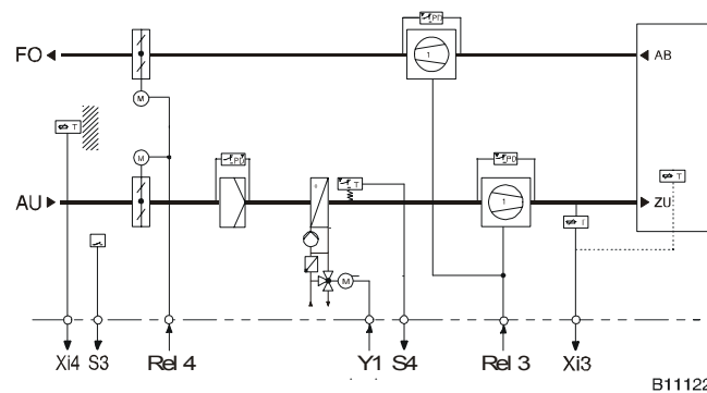
MOD 201: Пост. упр. (комн.-)тем. приточ. возд. с управл. вентилятором и заслонкой вентиляции
