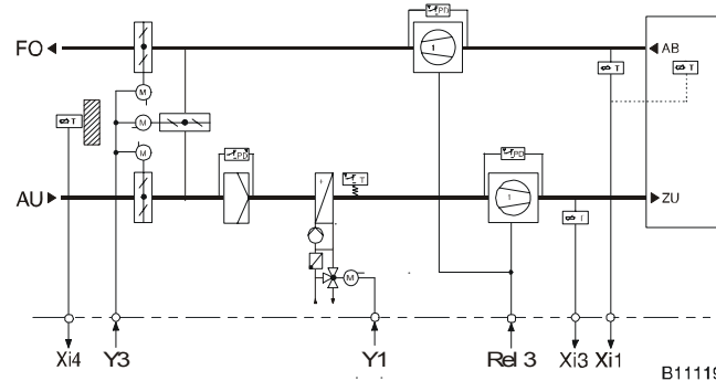
MOD 203: Каскадное упр. вытяжн.(комн.)/приточн. воздухом с рециркуляцией воздуха и нагревателем
